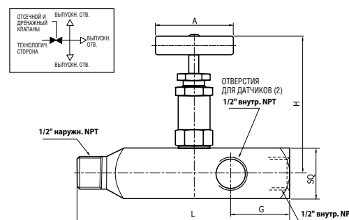
V46GR. Манометрический клапан
