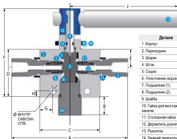
2-ходовой шаровой клапан
